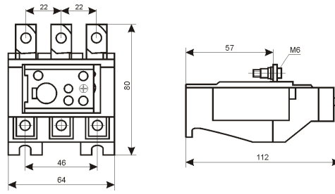
Рис. 1 Габаритные размеры PTT12-63
